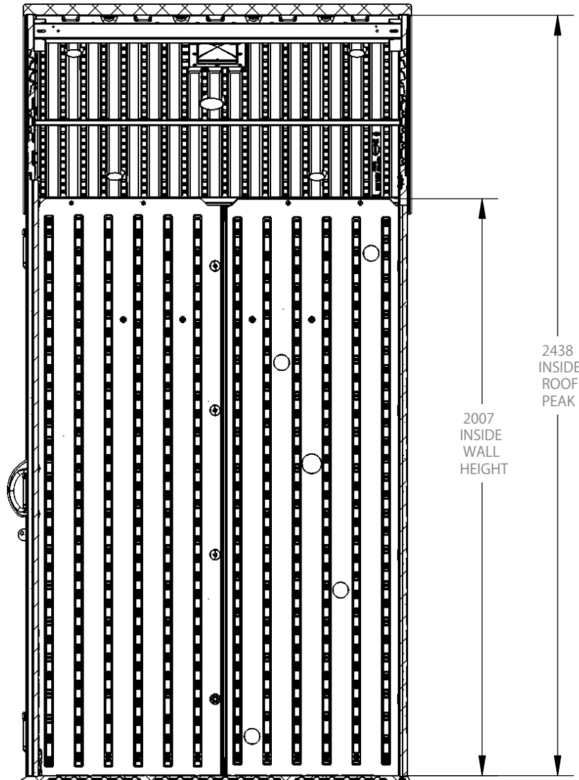
SECTION A-A SCALE 1:16
